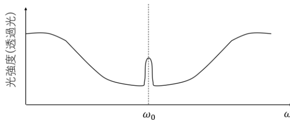
図 3 飽和吸収分光法 ラムディップ
