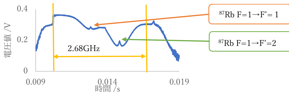
図5 吸収信号
