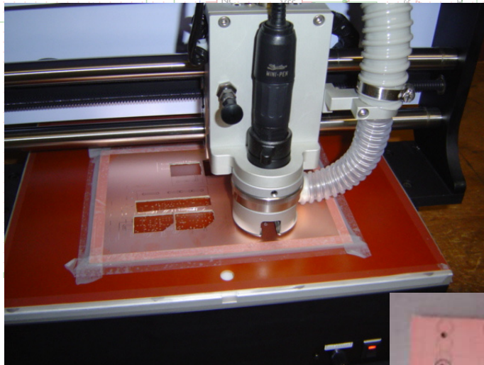
↑ 基板加工機
