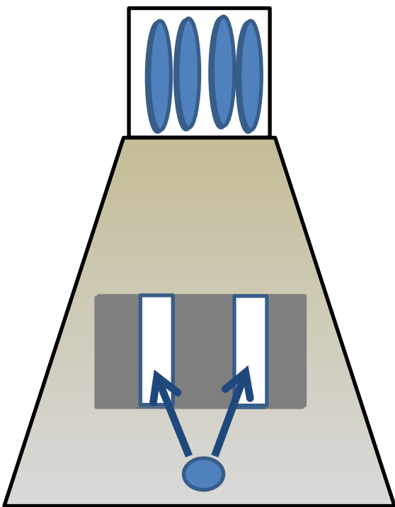
光子
